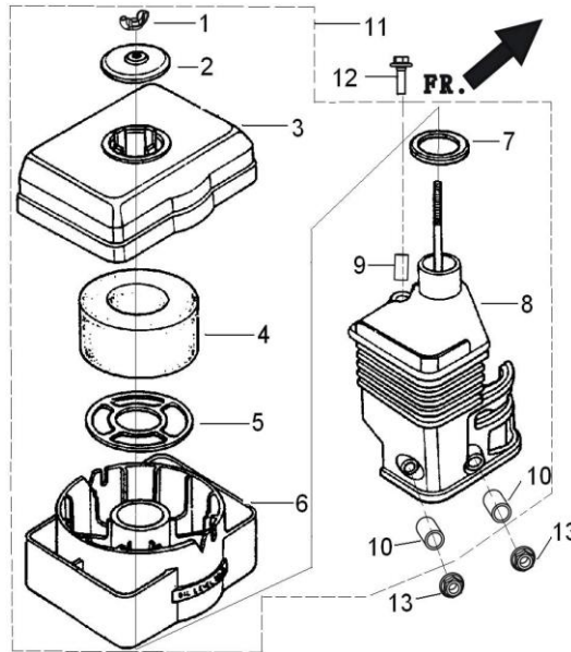
FIG.10 FILTRO DE AIRE EN BAÑO DE ACEITE ( F02 )
