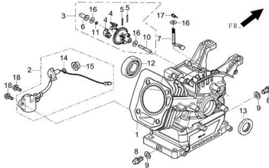
FIG.2 BLOQUE MOTOR (E17)
